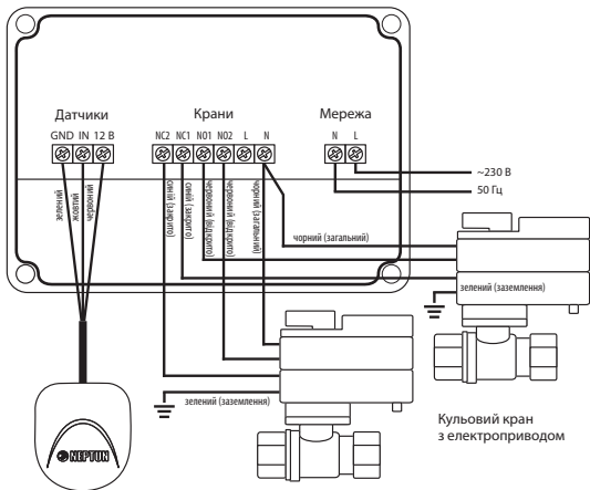
Мал. 2 Схема підключення кульового крану з приводом до модуля керування Neptune Base
