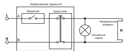
Рис. 6. Схема електрична
