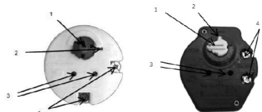
Рис. 3. Зовнішній вигляд терморегулятора 1.Повзун регулювання температури. 2.Кнопка теплового захисту. 3.Гнізда підключення сигнальної лампи. 4.Клеми підключення до електроенергії.
